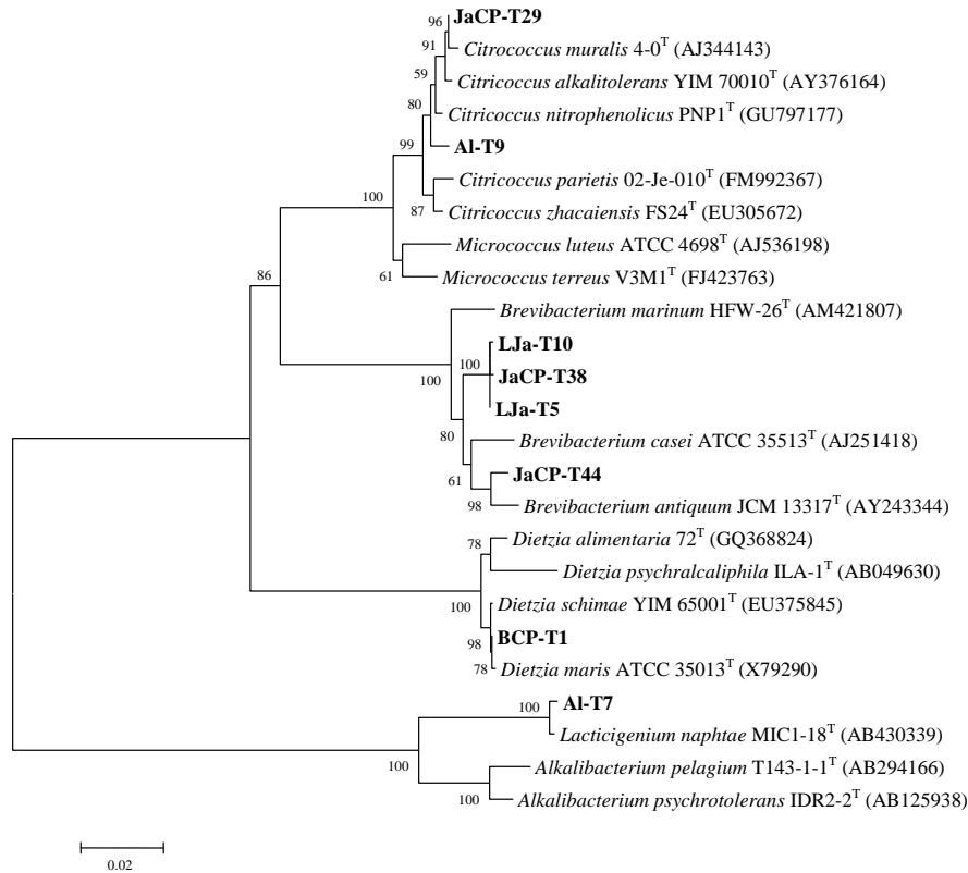
Рис. 1 Филогенетическая дендрограмма, построенная на основе анализа нуклеотидных последовательностей генов 16S рРНК некоторых штаммов, выделенных из арктических криопэггов, с использованием метода поиска ближайших соседей (“ neighbour-joining ”). Данные “bootstrap”-анализа (выраженные в процентах от 1000 реплик) указаны в точках ветвления.
